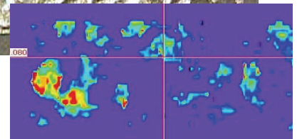
ACTUAL UT SCREEN OF EDM COUPON
